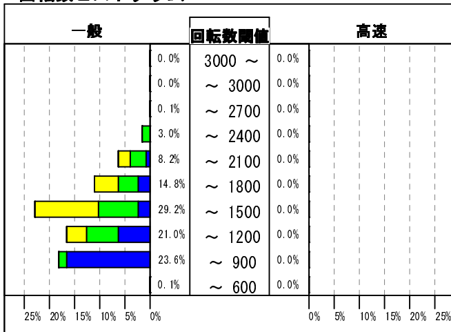
回転数ヒストグラム
