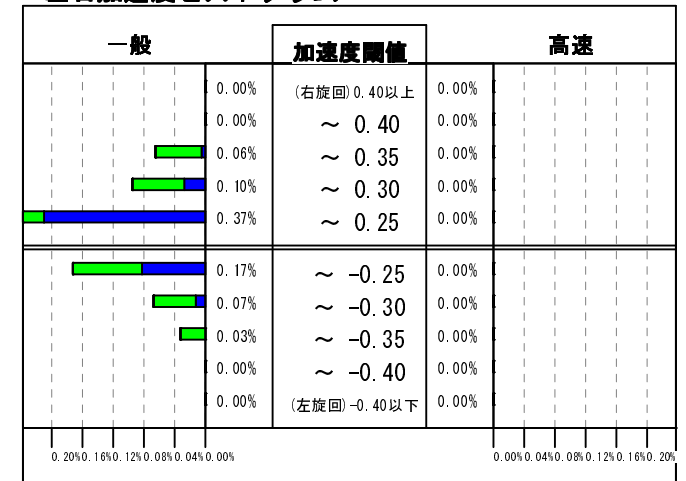
左右加速度ヒストグラム
