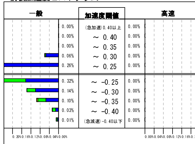
前後加速度ヒストグラム
